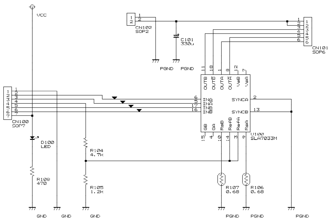
モータ接続例
