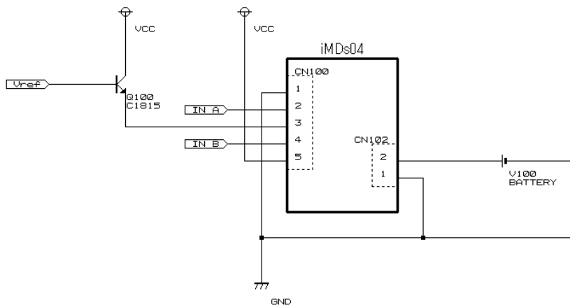
Fig. 4 マイコンからの電流値設定例
