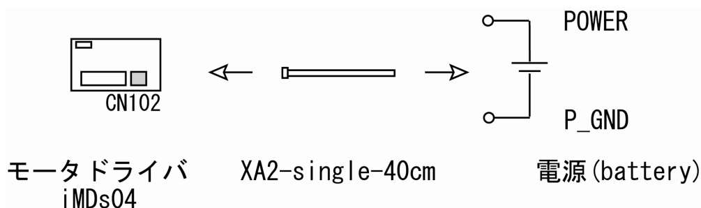
Fig. 5 モータ用電源との接続
