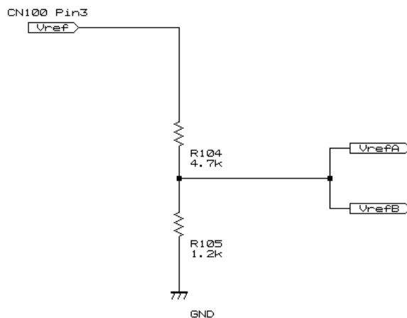
Fig. 3 電流設定信号
