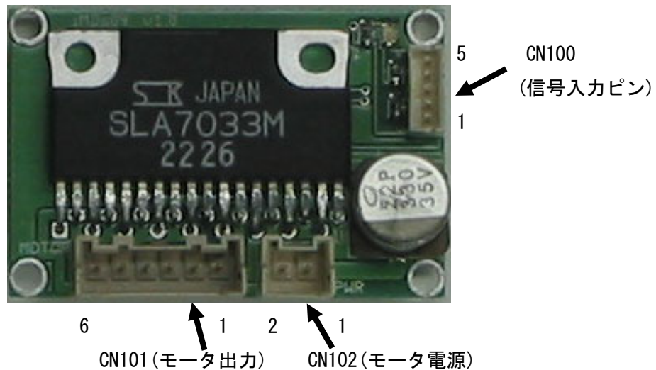
Fig.1 各部の名称
