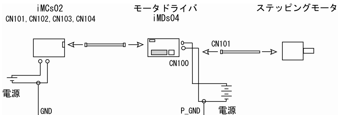
Fig. 6 GND 接続例
